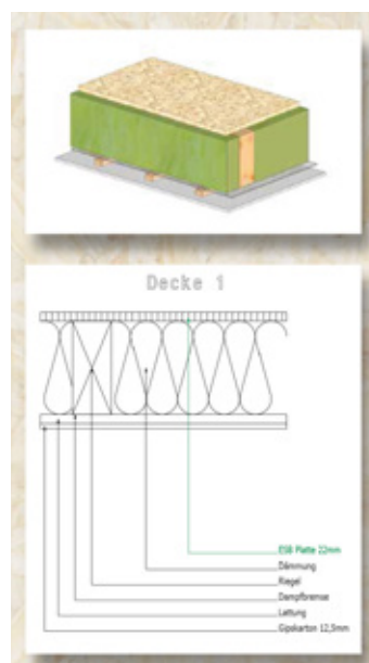
Aufbau oberste Geschossdecke beim Kaltdach
