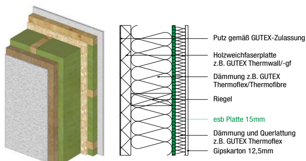
Außenwand 3 – mit Wärmedämmverbundsystem Holzfaser
