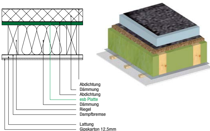
Abbildung 4 – Nicht belüftetes Flachdach mit Zusatzdämmung oberhalb der Tragkonstruktion
