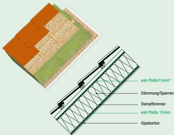
Dach 1 – esb-Platte mit hoher aussteifender Wirkung
