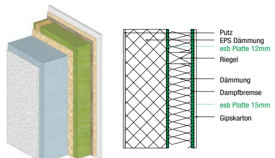
Außenwand 4 – mit Wärmeverbundsystem EPS
