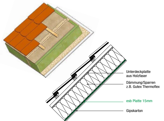
Dach 2 – Unterdeckplatte aus Holzfaser ohne aussteifende Wirkung
