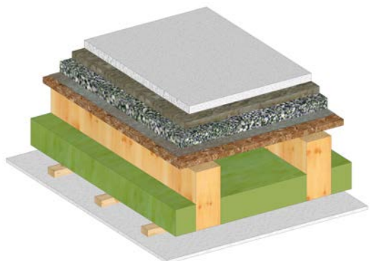
Innendecke 3 – zum beheizten Raum
