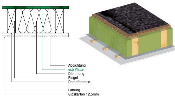
Abbildung 3 – Nicht belüftetes Flachdach mit Volldämmung in der Tragebene
