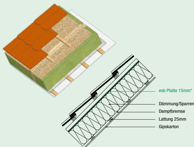
Dach 3 – esb-Platte mit hoher aussteifender Wirkung
