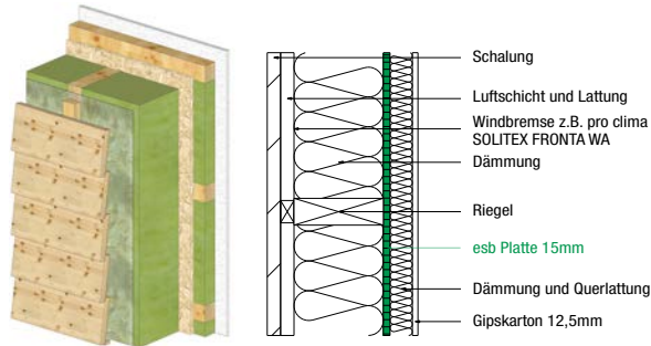
Außenwand 1 – hinterlüftet
