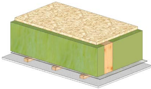
Innendecke 1 – zum unbeheizten Raum
