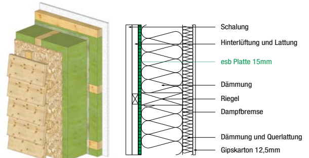
Außenwand 2 – hinterlüftet
