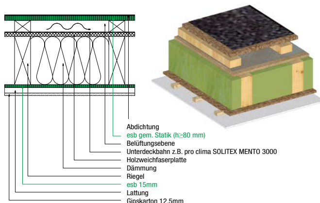
Abbildung 2 – Volldämmung mit unterlüfteter Dachhaut
