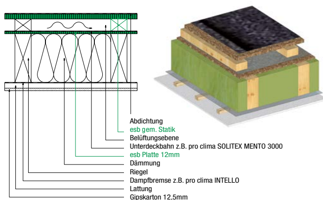
Abbildung 1 – Flachdach mit unterlüfteter Dachhaut
