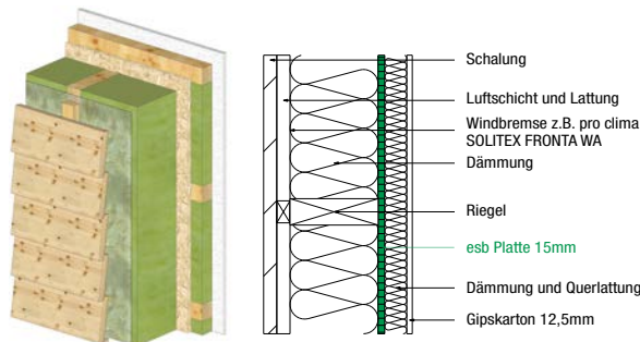
Außenwand 1 – hinterlüftet
