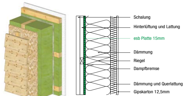
Außenwand 2 – hinterlüftet
